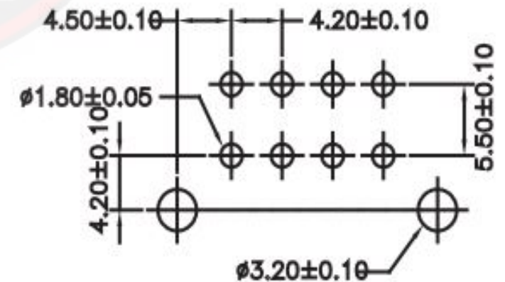
P.C.B LAYOUT
