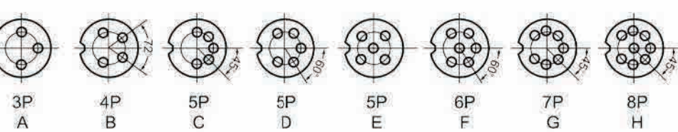
YY7006 DIN chassis plug (3P-8P)
