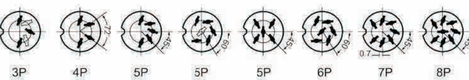
YY7007 DIN jack (3P-8P)
