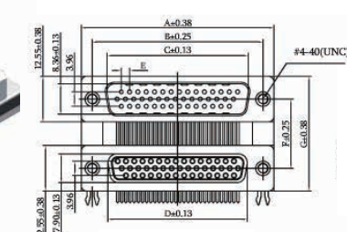
P/N: 317-6-4128-XX
