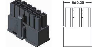
P/N:517-9-45-XX
