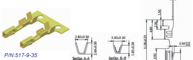
P/N:517-9-35
