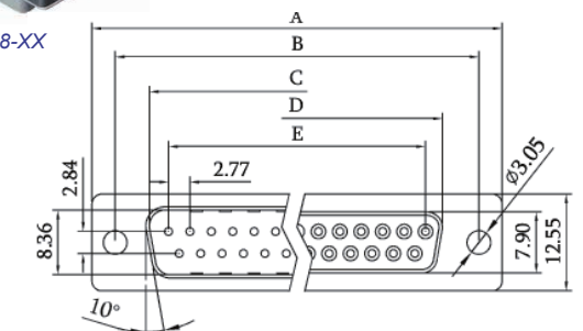
P/N: 317-6-4129-XX
