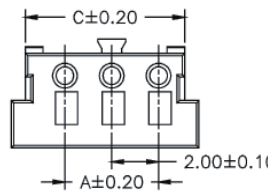
P/N:517-9-24-XX
