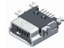
P/N:517-3-0129
