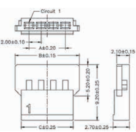
P/N:517-9-28-XX
