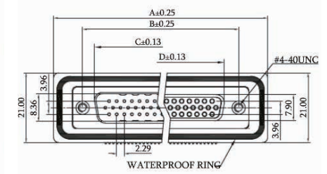
P/N: 317-6-4126-XX
