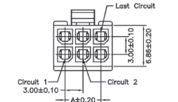
P/N:517-9-45-XX
