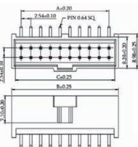
P/N:517-9-43-XX
