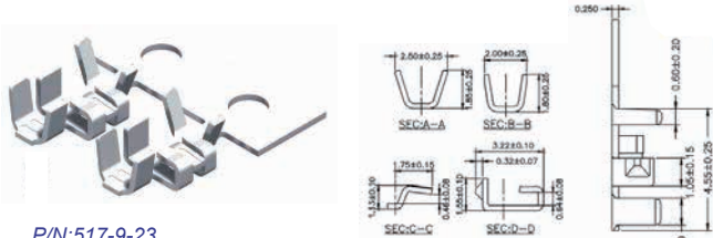
P/N:517-9-23
