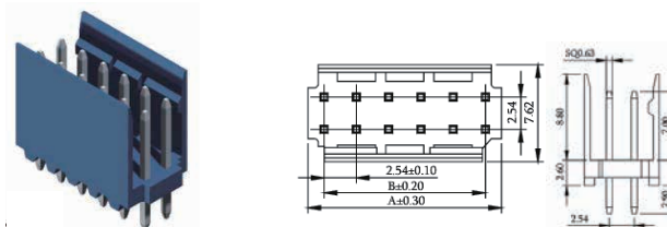
P/N:517-9-32-XX
