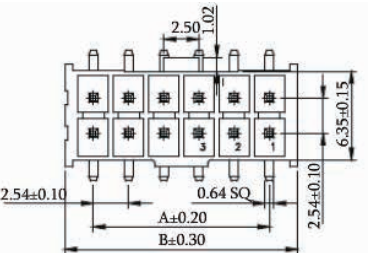
P/N:517-9-38-XX
