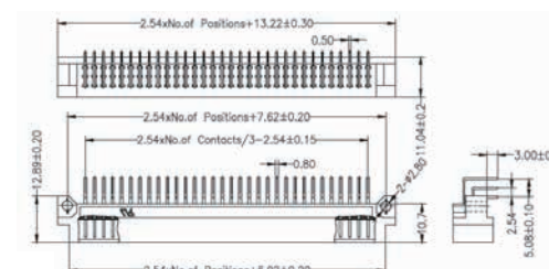
P/N: 517-15-2001
