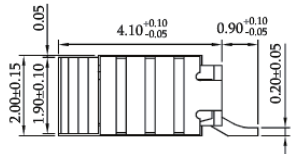
P/N:517-10-18-XX
