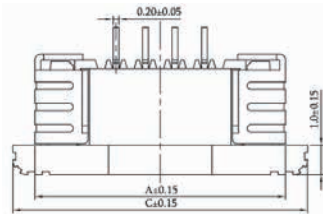
P/N:517-10-16-XX
